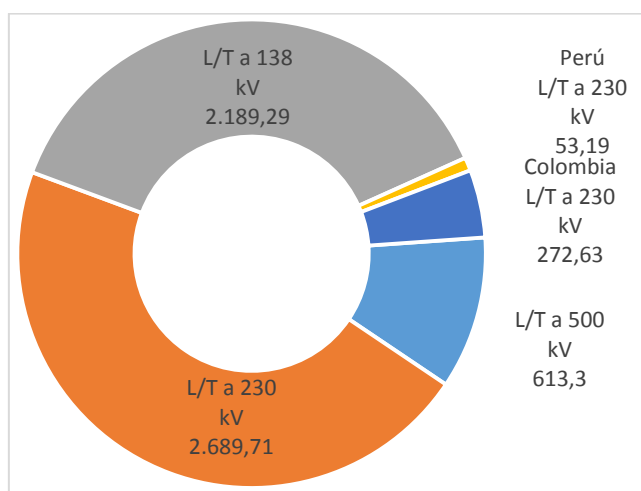
Figura Nro. 5-2: Composición y longitud en km de líneas de transmisión del SNT.
