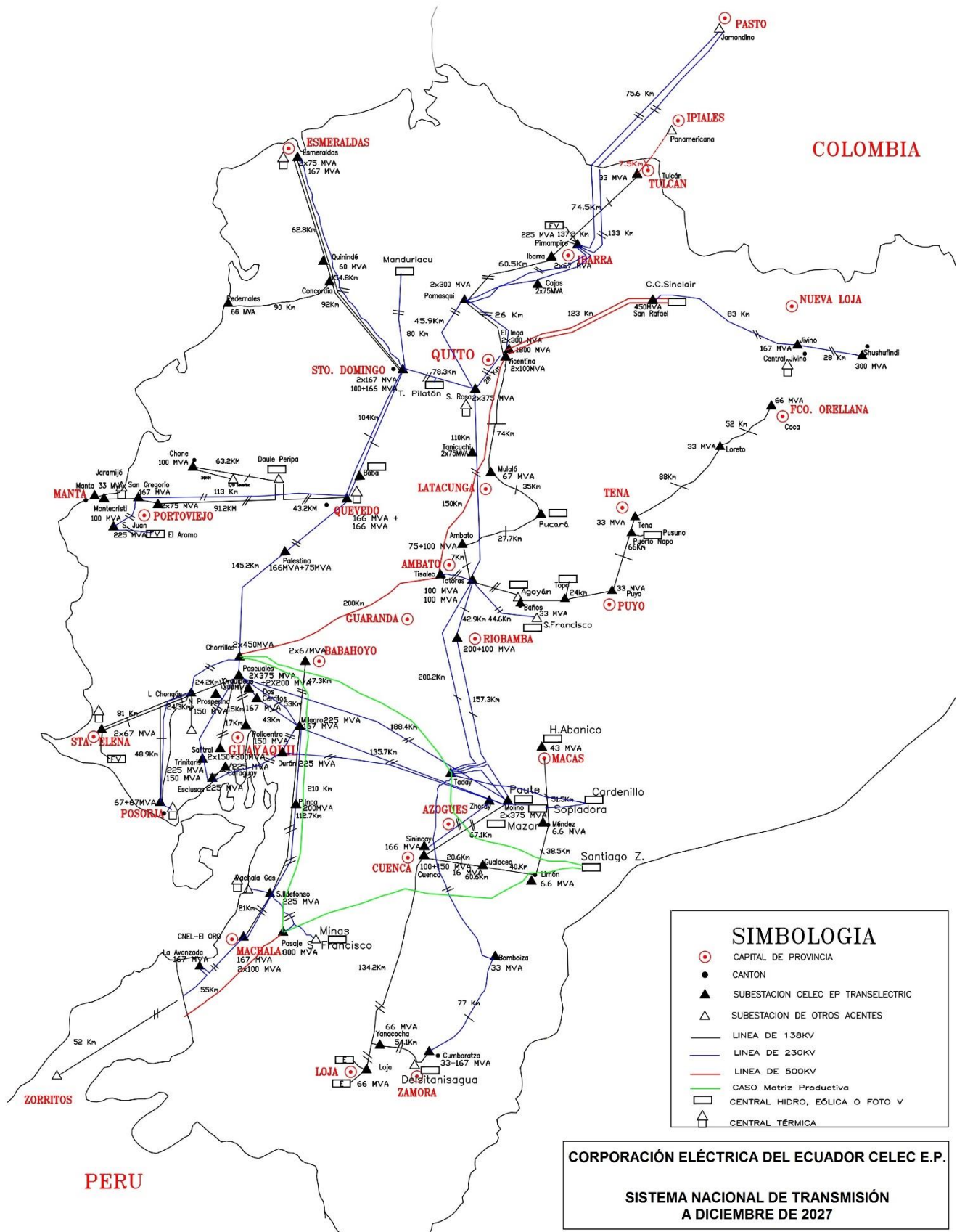
Figura Nro. 5-6: Esquema geográfico del Sistema Nacional de Transmisión – Año 2027
