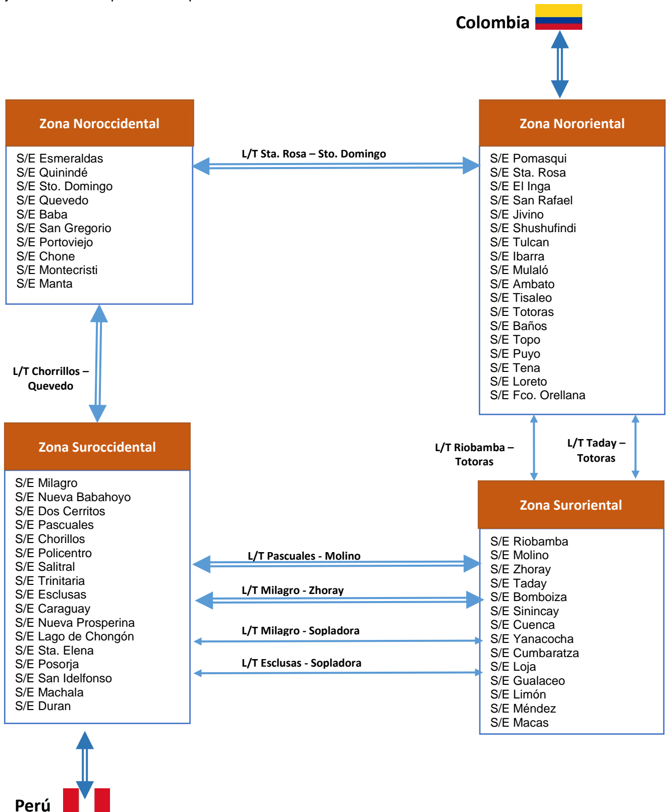
Figura Nro. 5-3: Subestaciones y zonas operativas del SNT
