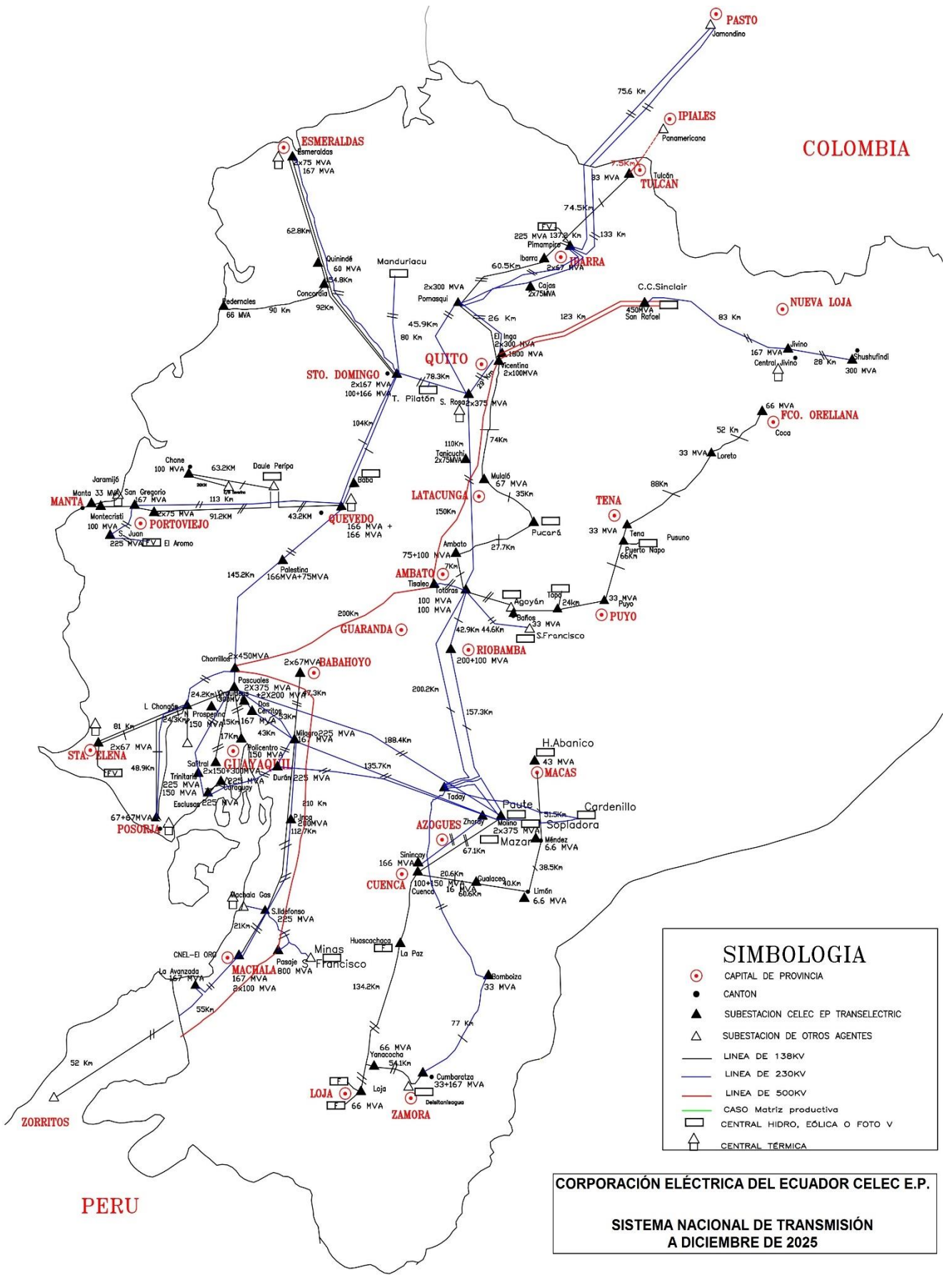
Figura Nro. 5-5: Esquema geográfico del Sistema Nacional de Transmisión – Año 2025
